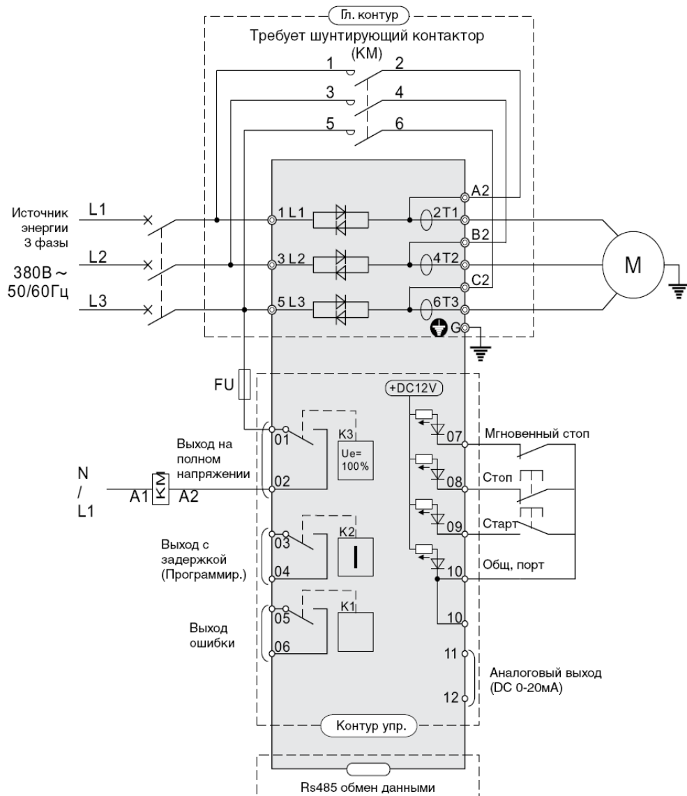
Рисунок 2-3-1 Схема подключения
