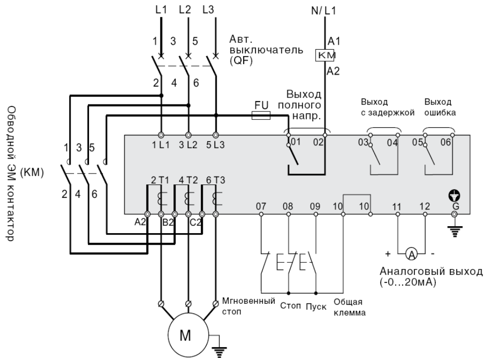
2-9 Схема подключения реле и пульта управления
