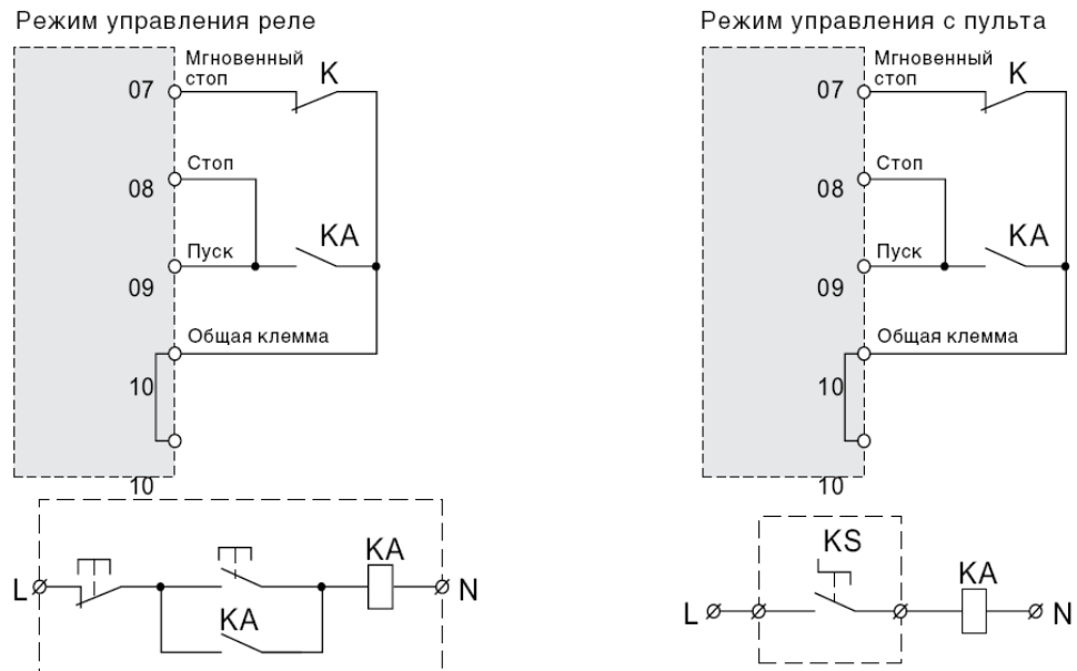
2-9 Схема подключения реле и пульта управления
